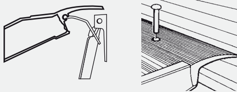
A- Zungenauflager
