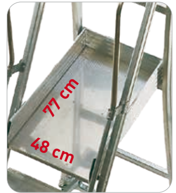
Plate-forme en tôle d'aluminium
