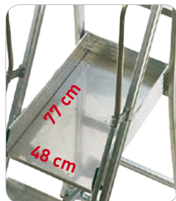
Plate-forme en tôle d'aluminium
