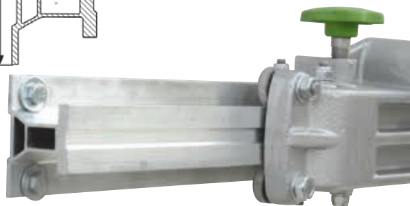
Chariot composé de 12 coussinets et 2 vis de blocage
