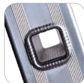
Echelon carré: 30 x 30 mm solidement bloqué aux montants
