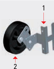
1-PORTA RUOTA SOLLEVABILE IN ACCIAIO (PINNA) SENZA RUOTA
