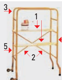
1- coppia assi Cod. LE-002
