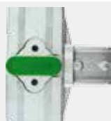
RACCORDO A CROCERA IN FUSIONE PER TRAVERSA (CON TIRANTI A MOLLA) Cod. D823
