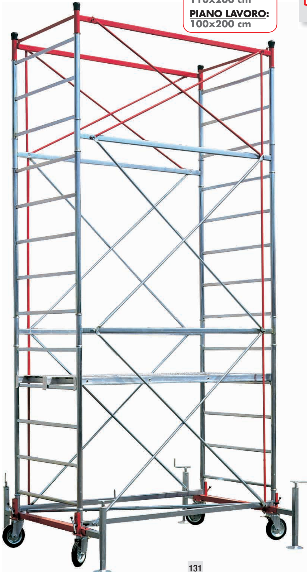
Protezioni terminali
