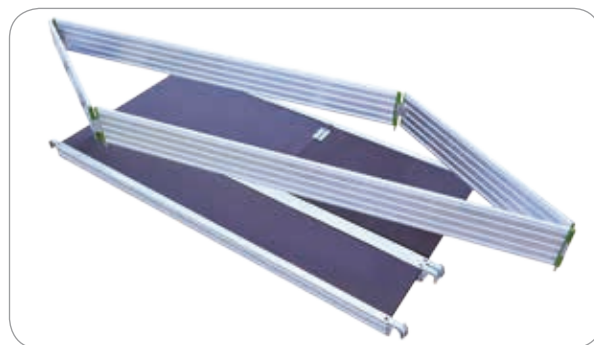
Plateau: structure en aluminium avec surface en bois Eurodeck antidérapant et résistant à l'eau.
