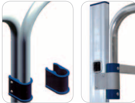
Klapp-Rahmenteil Gelenk. Nylon Buchse für Gelenk.
