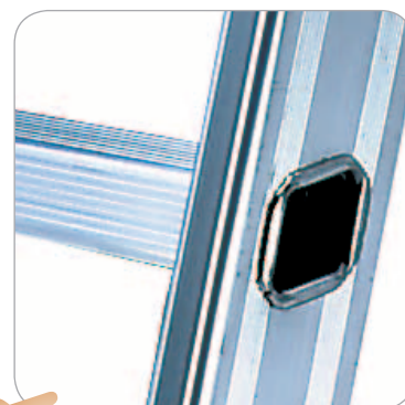
Hochfeste FACAL-Profi-Verbördelung 30x30 mm, rhombisch eingebaut für optimalen Stand.
