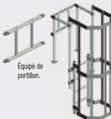
MODULE TERMINAL AVEC GARDE-CORPS ET PORTILLON (pattes de fixation non comprises)
