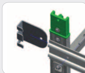
Patte de fixation crinoline / échelle
