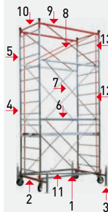
6- TRAVESSA LATERALE Cod. ST
