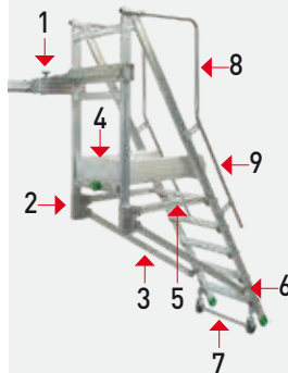
SOLO VOLANTINO C/INSERTO PER CARRELLO
