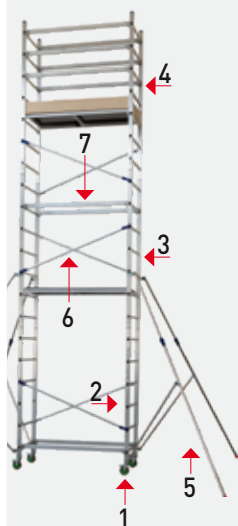
3- SOLO SPALLA A 7 GRADINI MODULO 2 Cod. AL-SP7M2
